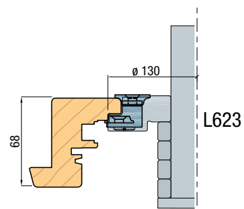
Draaikiep opdek 17 mm stolp met dubbele kierdichting
