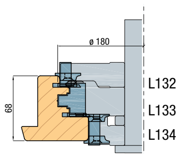
Draaikiep opdek 17 mm stolp met dubbele kierdichting — passief raam
