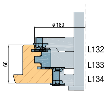
Draaikiep opdek stol met dubbele kierdichting — passief raam
