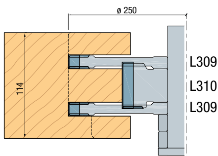
Slissen met contra kalkspinning opdek
