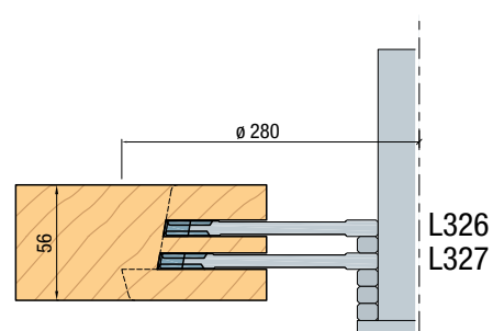
Slissen ramen buitenbeglazing
