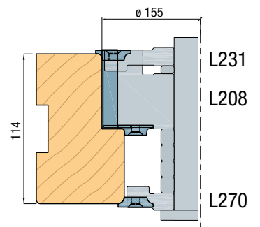
Bovendorpel / stijl
