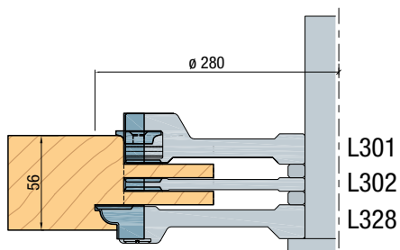
Dubbele pen ramen
