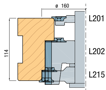
Stijl met scharniersponning
