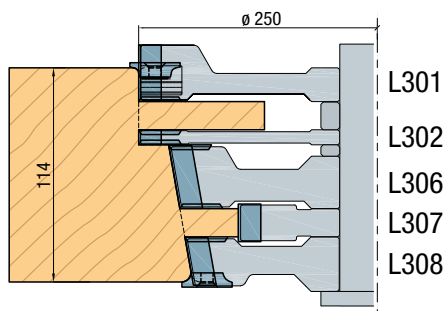
Contra onderdorpel
