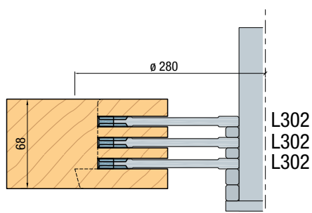
Slissen ramen 3 vlaks
