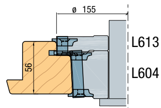
Ramen met kaderdichting stijl en bovendorpel
