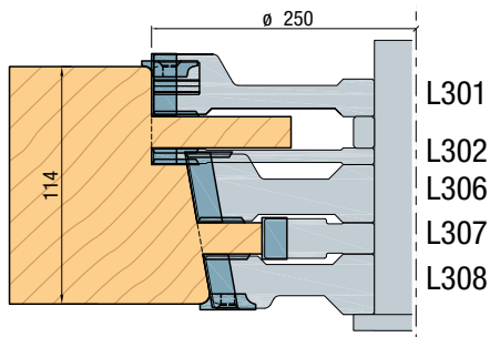
Contra onderdorpel
