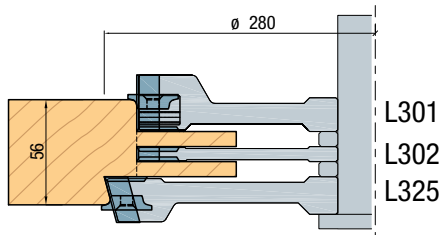
Dubbele pen ramen
