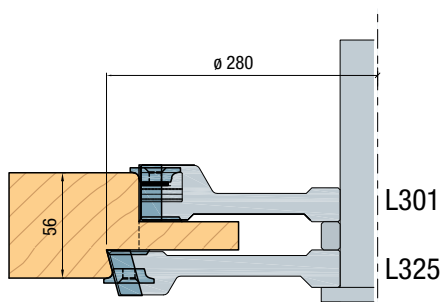
Enkele pen deuren 56 mm
