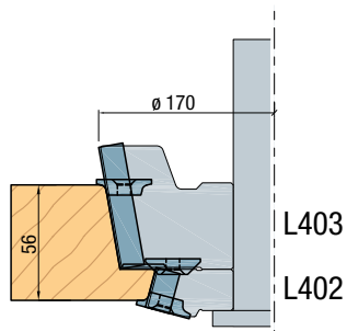
Slissen ramen buitenbeglazing
