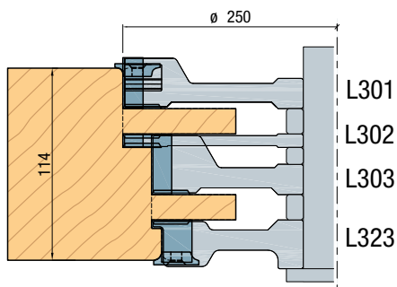
Contra stijl / kalf
