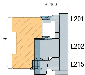
Stijl met scharniersponning
