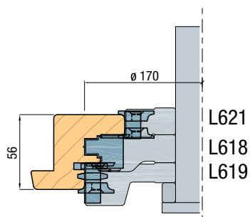
Draaikiep opdek onderdorpel
