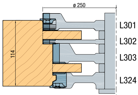
Contra bovendorpel
