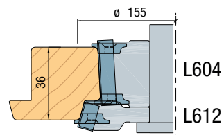
Ramen met kaderdichting stijl en bovendorpel
