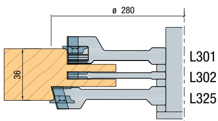
Dubbele pen ramen
