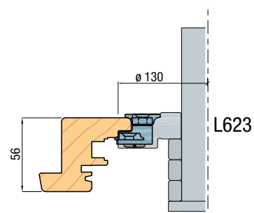
Draaikiep stolp met dubbele kierdichting
