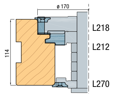
Tussendorpel kalf — stijl
