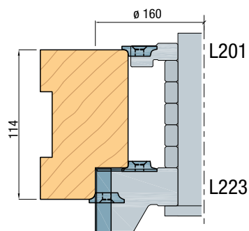
Stijl - bovendorpel onderdorpel stomp
