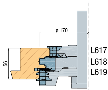
Draaikiep Contura onderdorpel
