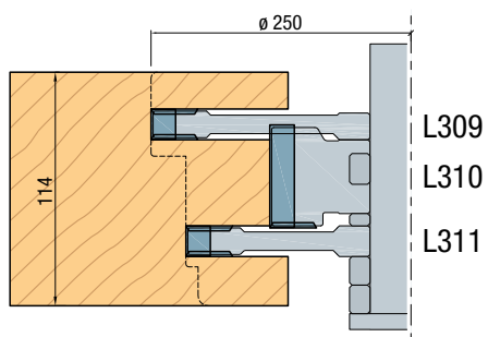
Slissen met contra kalksponning
