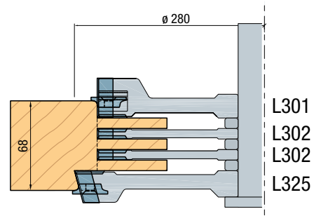
Pennen ramen 3 vlaks
