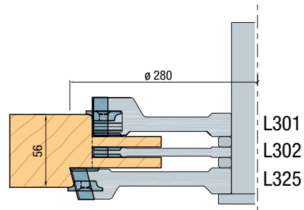
Dubbele pen ramen 56 mm
