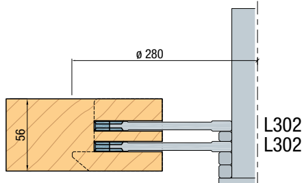
Slissen ramen
