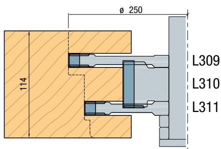
Slissen met contra kalksponning
