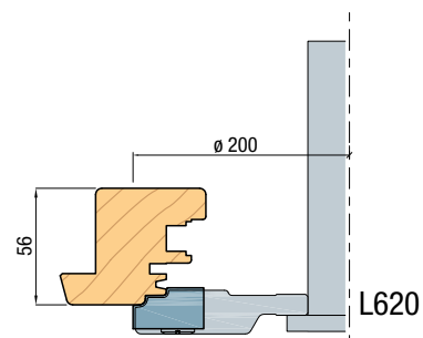
Draaikiep Contura onderdorpel
