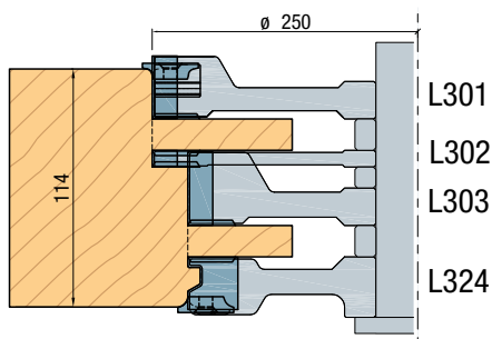
Contra bovendorpel
