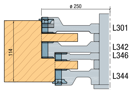
Contra stijl / kalf bovendorpel onderdorpel stomp
