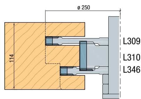
Slissen met contra kalkspinning stomp
